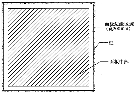
图3 门窗、幕墙各部件划分示意图
